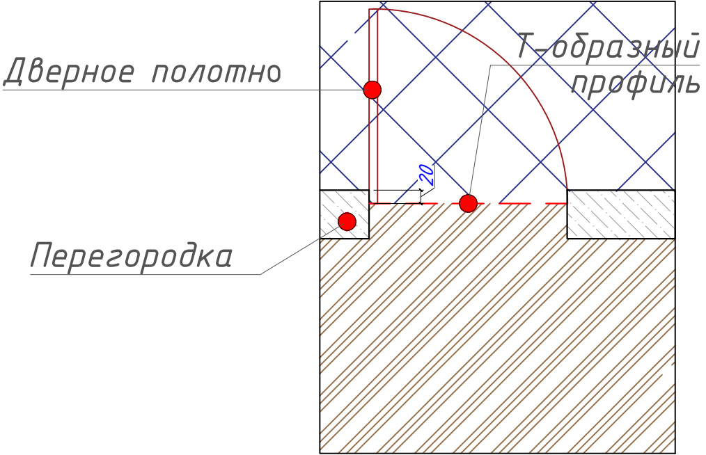
Узел 1
