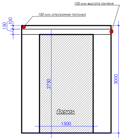
Развертка 1
