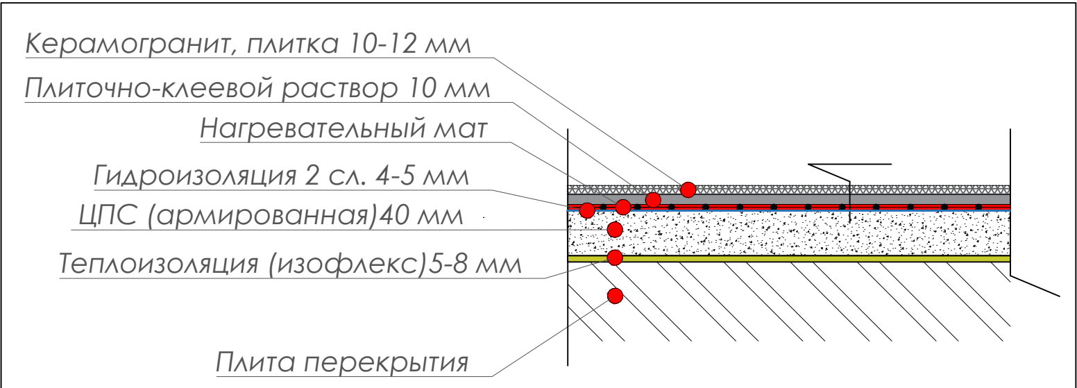
Конструкция пола 2
