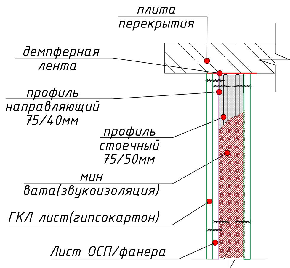
Сечение 1-1
