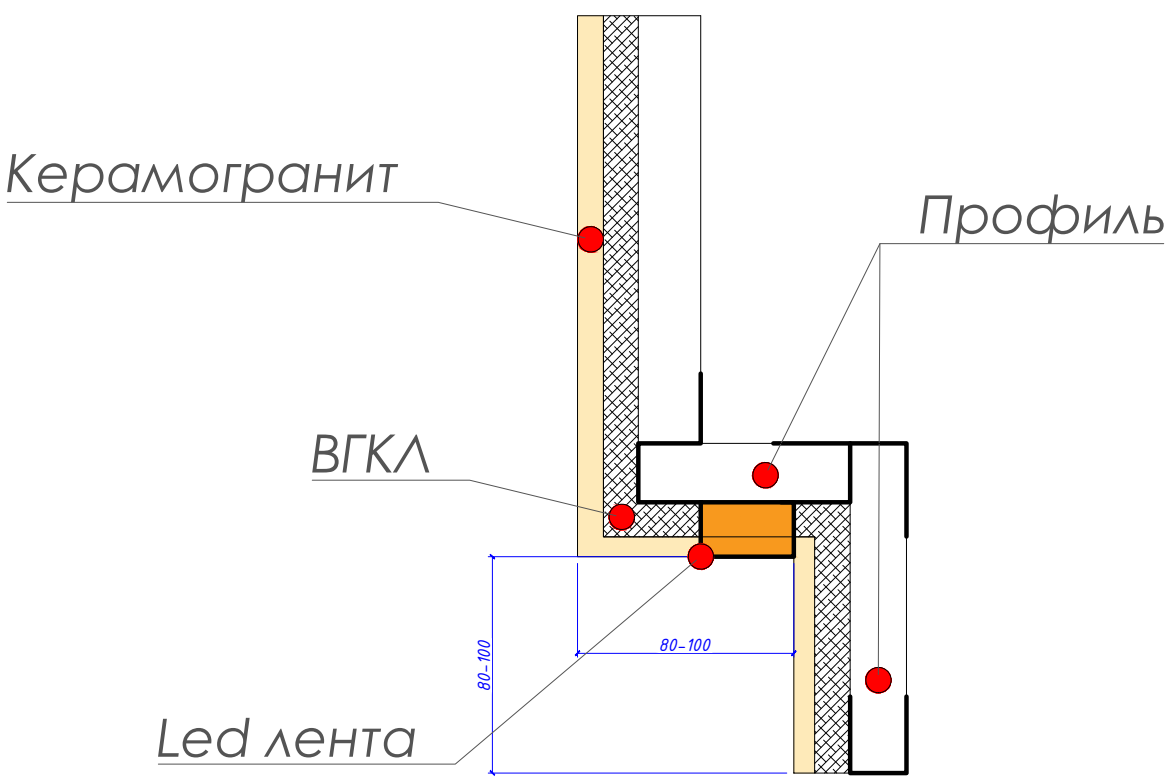
Сечение 2-2 НИША ДЛЯ НОГ В ВАННОЙ С ПОДСВЕТКОЙ
