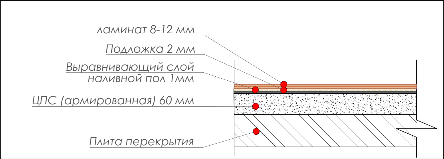
Конструкция пола 1
